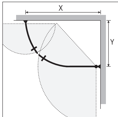
Vänsterhängd dörr
