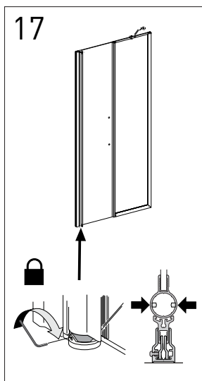
17 Dörrrens stängningsläge bestäms av positionsbrickan. Lås positionsbrickan med dess två låsskrivar i önskat läge.
