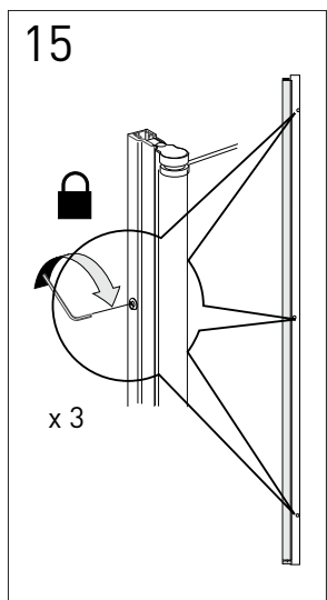
15 Lås dörrbladet vid vägprofilen med vägprofilens tre spännskravar. Spännskravarna skall efterdras efter ca 14 dagars användning.
