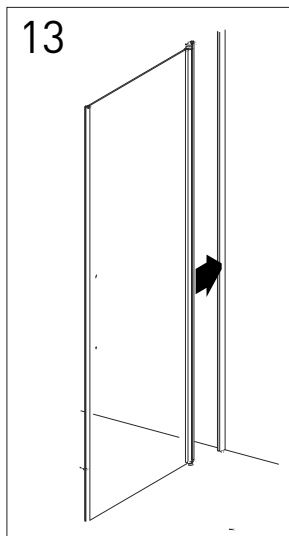
13 Tryck fast dörrbladet i vägprofilen. Säkerställ att dörren är rättvänd.
