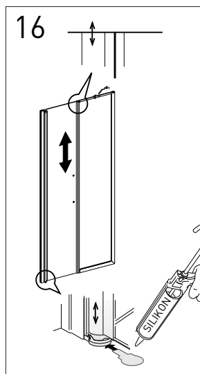
16 Dörrbladens överkant skall linjera. Justera vid behov genom att använda de gitarrformade distansklossarna. Applicera silikon mellan golv och golvbestag. Används distansklossar skall silikon även appliceras på dessa.
