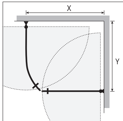
Vänsterhängd dörr
